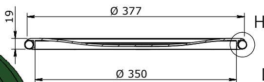
SEÇÃO G-G ESCALA 1 : 6.5
